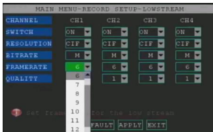
Рис. 56. Настройка небольшого битрейта
