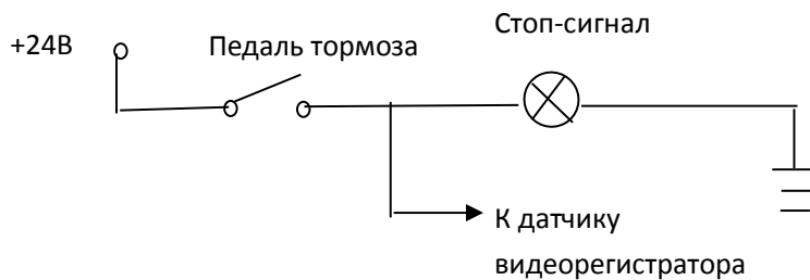
Схема для нажатия педали тормоза
