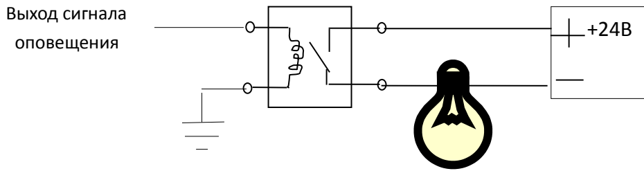
Схема подключения оповещающего устройства
