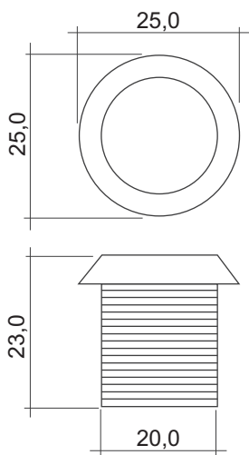
Рис.1 Габариты изделия.
