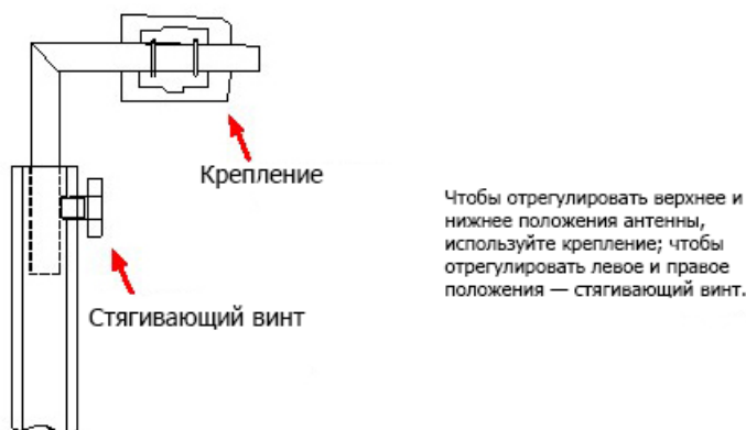
Рисунок 9. Монтаж крепления антенны.
