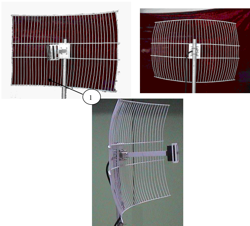
Рисунок 4. Внешний вид решетчатой антенны L-диапазона.
