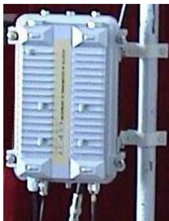
Рисунок 8. Внешний вид передатчика WS-0902.
